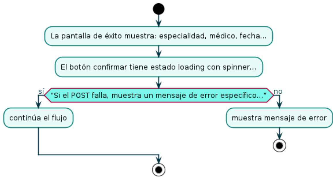
Diagrama de Estado — RF-22
