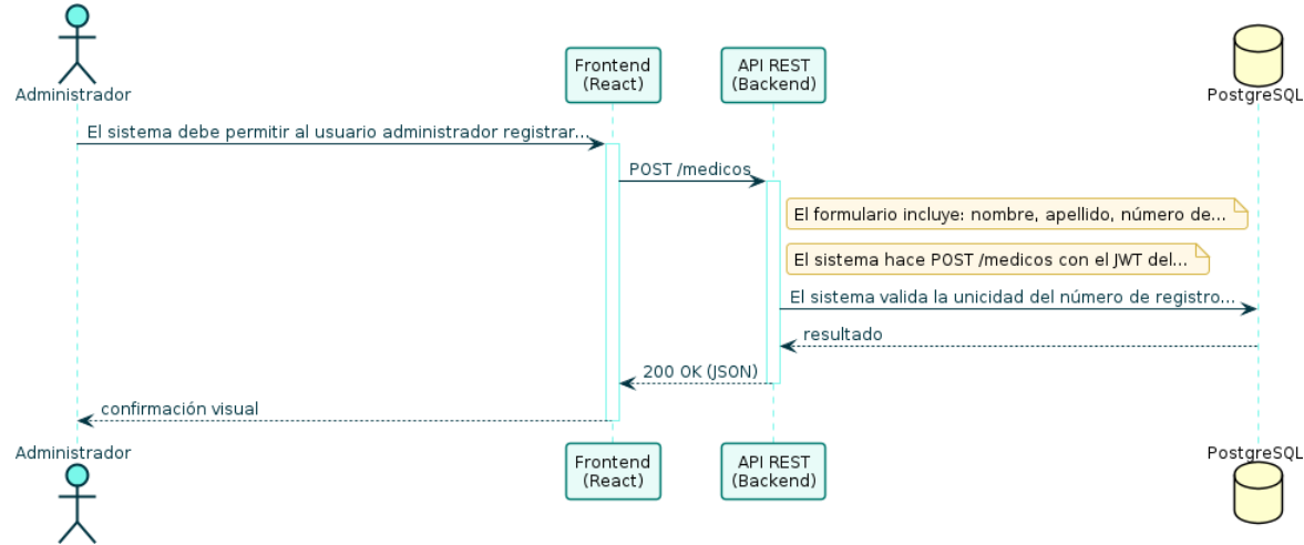
Diagrama de Secuencia — RF-33
