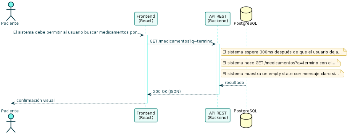
Diagrama de Secuencia — RF-25
