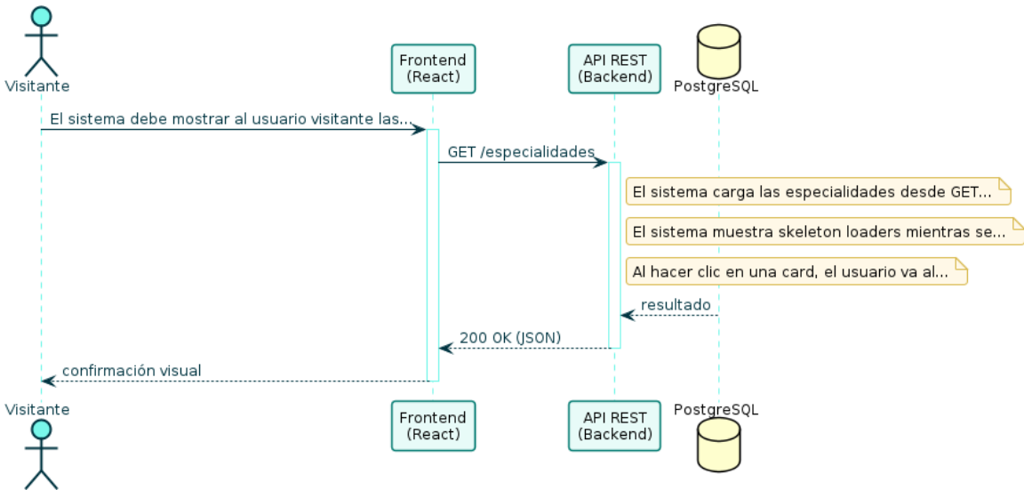
Diagrama de Secuencia — RF-08
