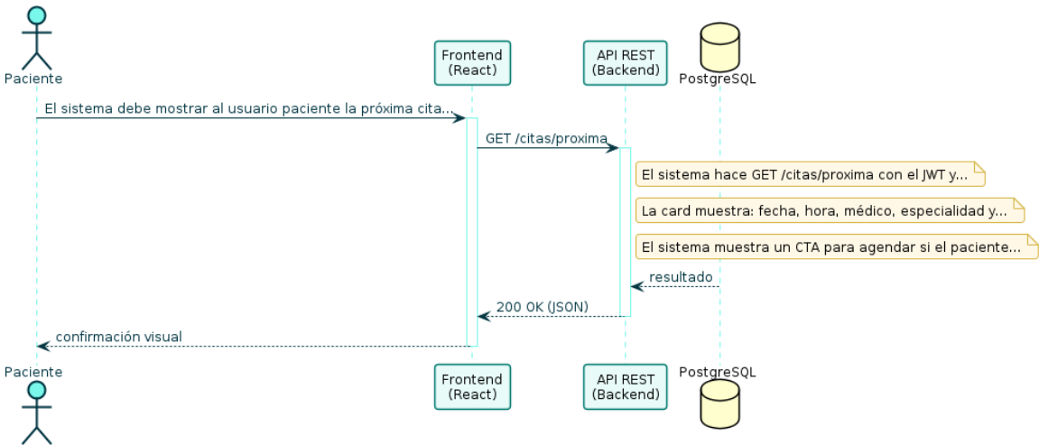
Diagrama de Secuencia — RF-41
