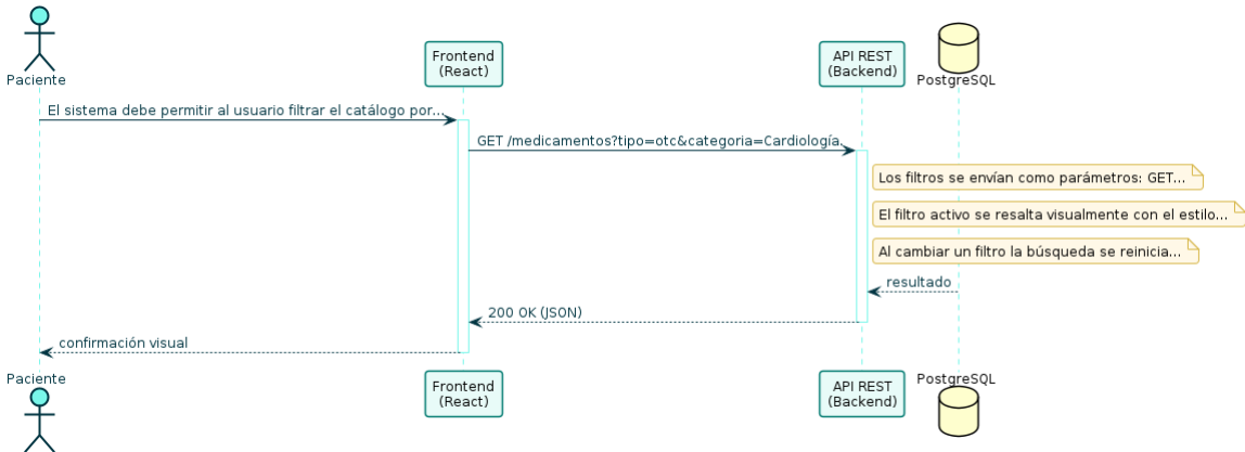
Diagrama de Secuencia — RF-26
