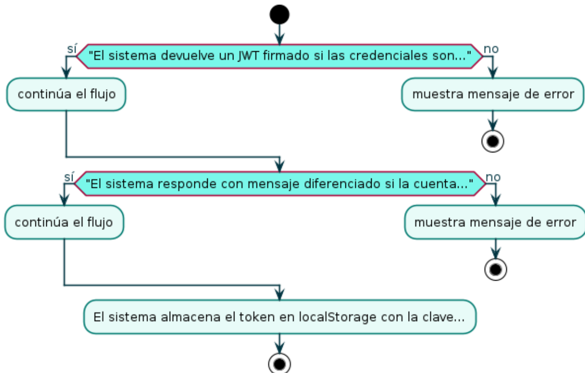
Diagrama de Actividades — RF-04
