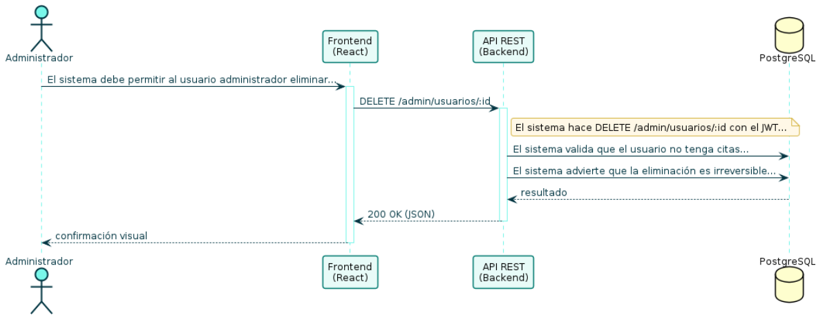
Diagrama de Secuencia — RF-50
