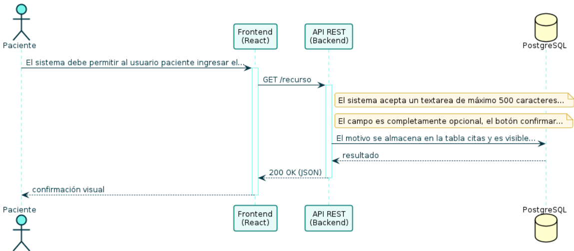
Diagrama de Secuencia — RF-20
