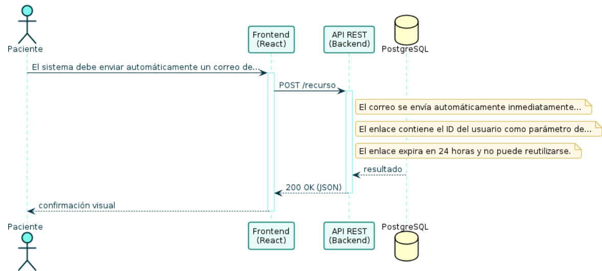
Diagrama de Secuencia — RF-02
