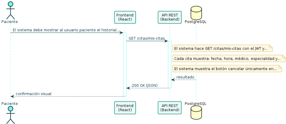
Diagrama de Secuencia — RF-38
