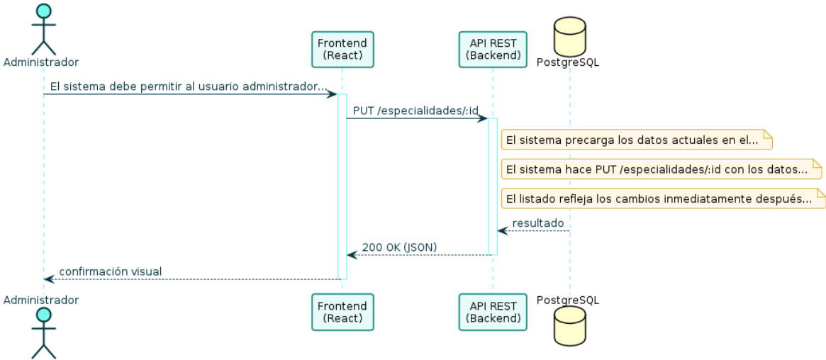
Diagrama de Secuencia — RF-14
