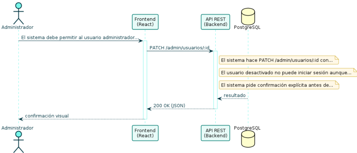
Diagrama de Secuencia — RF-49
