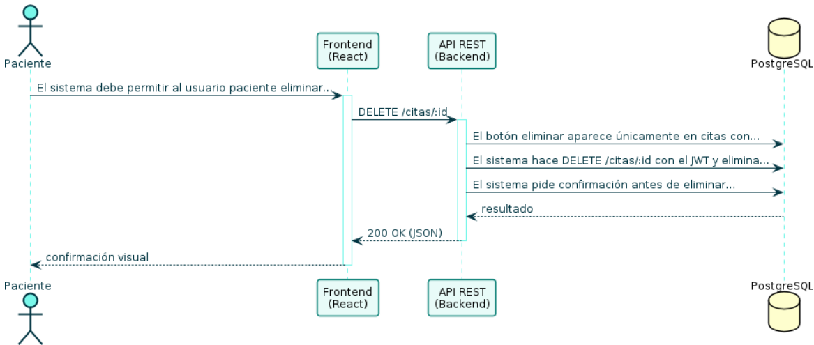
Diagrama de Secuencia — RF-40
