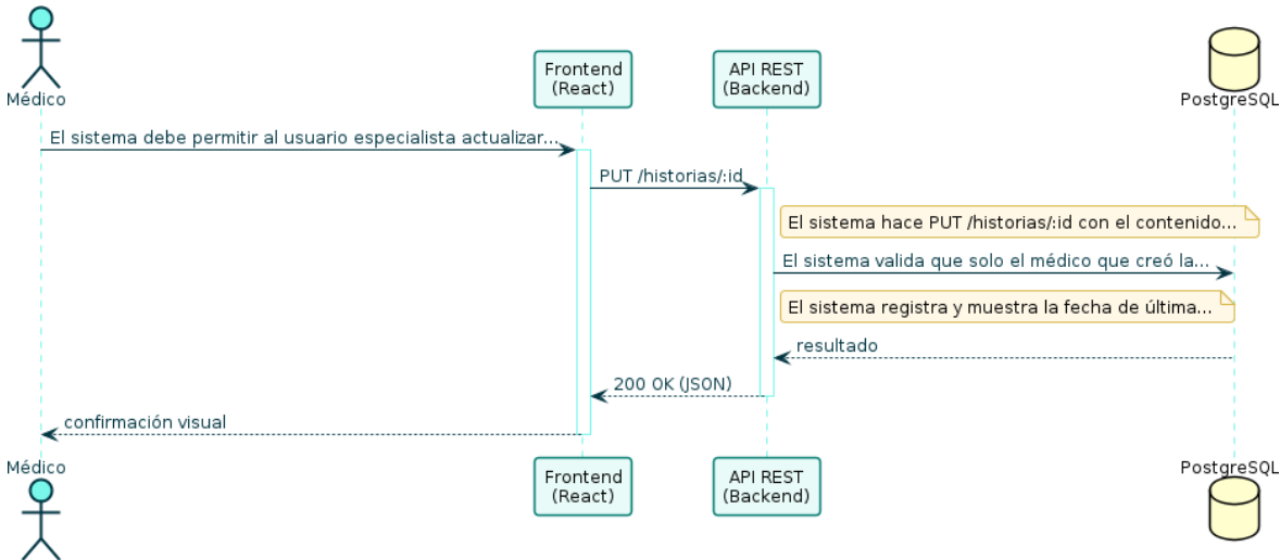
Diagrama de Secuencia — RF-46
