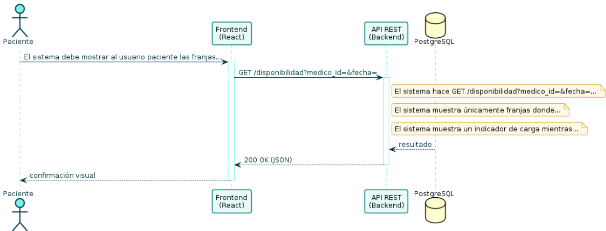
Diagrama de Secuencia — RF-17
