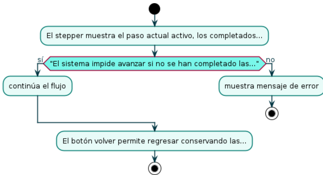
Diagrama de Estado — RF-16
