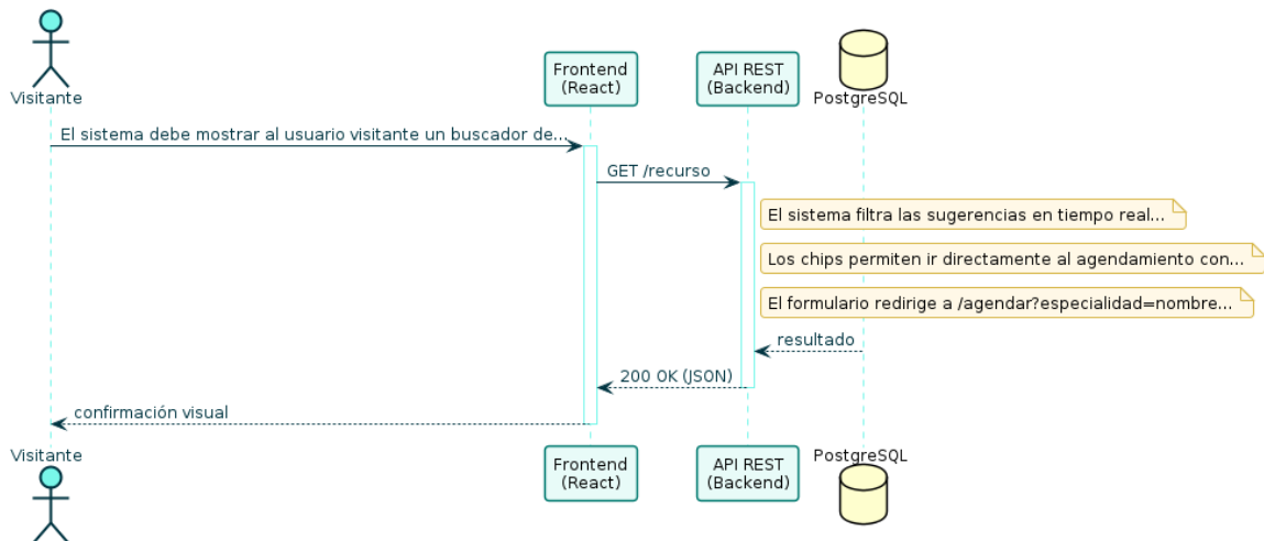
Diagrama de Secuencia — RF-07
