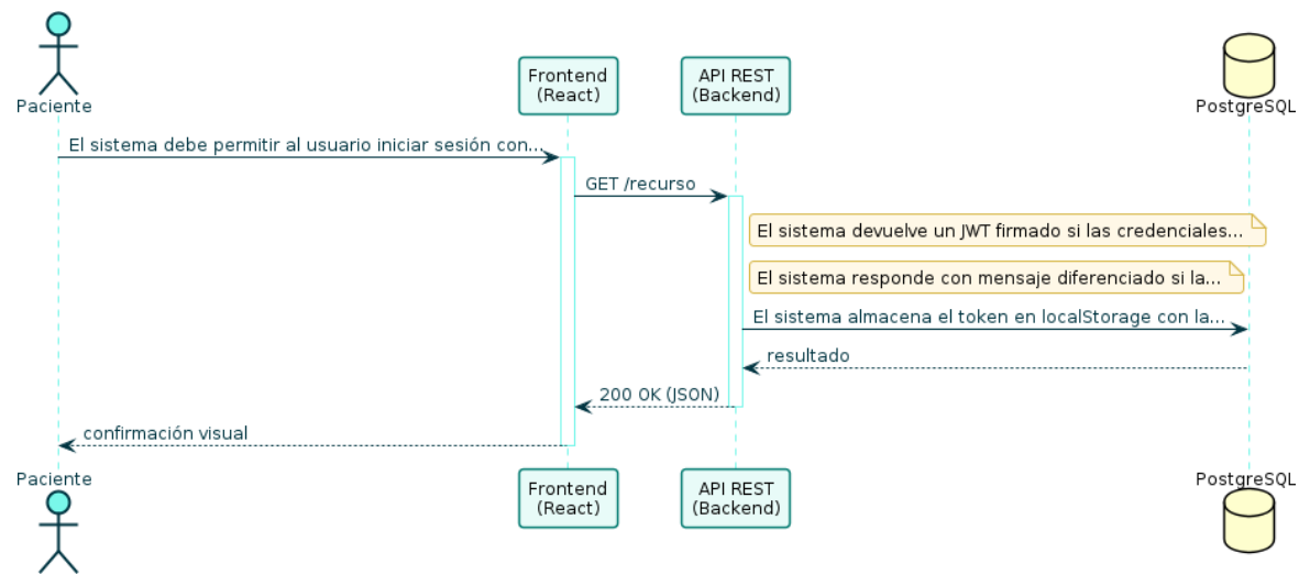
Diagrama de Secuencia — RF-04
