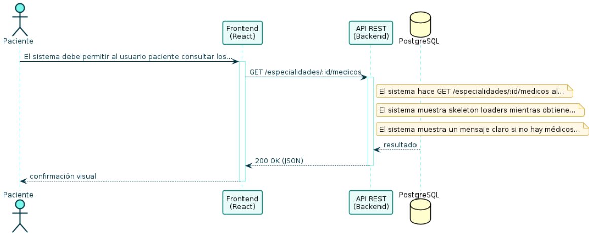
Diagrama de Secuencia — RF-12
