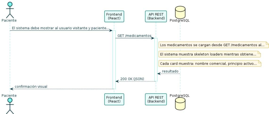
Diagrama de Secuencia — RF-24
