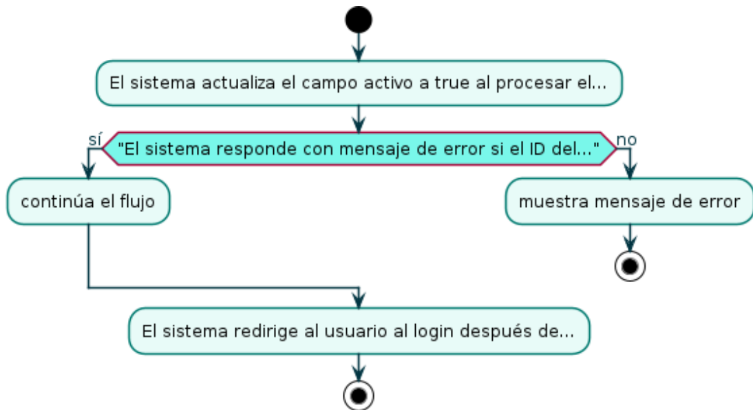
Diagrama de Actividades — RF-03
