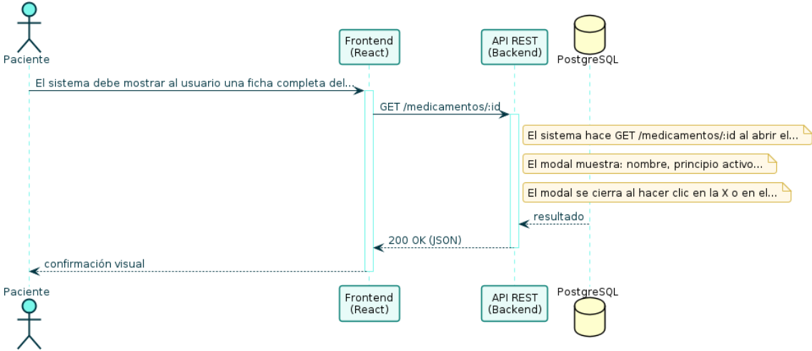
Diagrama de Secuencia — RF-27
