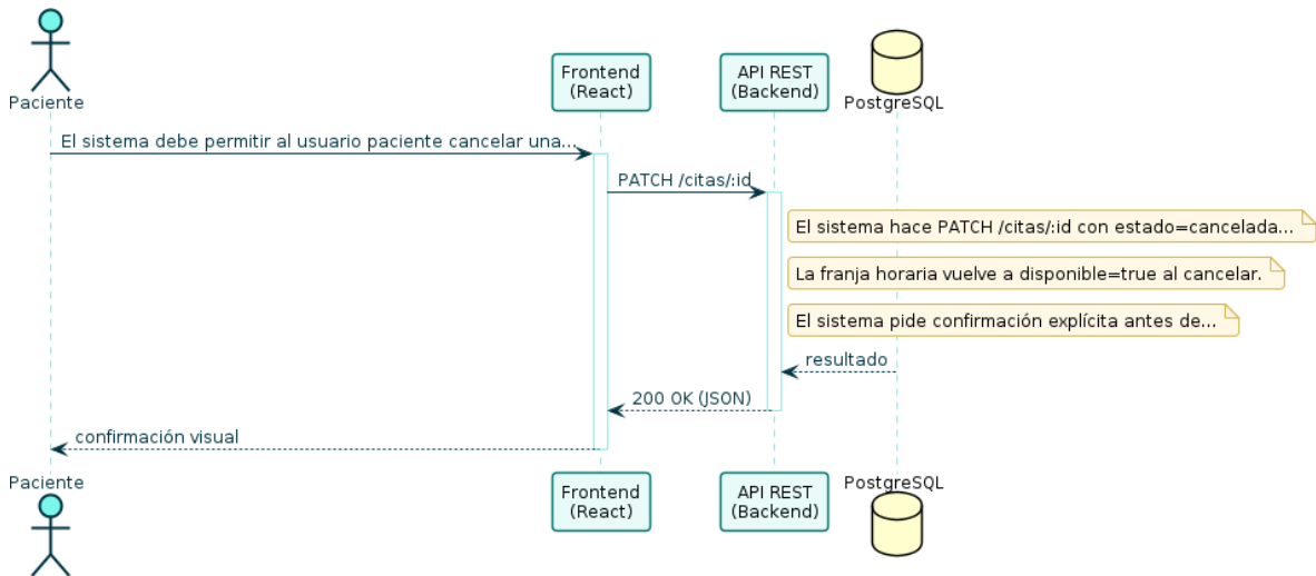
Diagrama de Secuencia — RF-23
