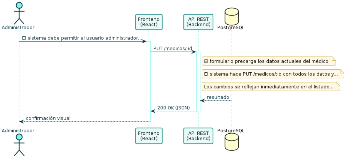
Diagrama de Secuencia — RF-34
