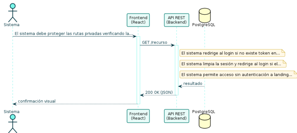
Diagrama de Secuencia — RF-06
