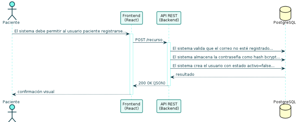
Diagrama de Secuencia — RF-01
