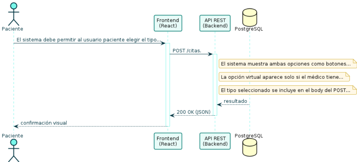
Diagrama de Secuencia — RF-19
