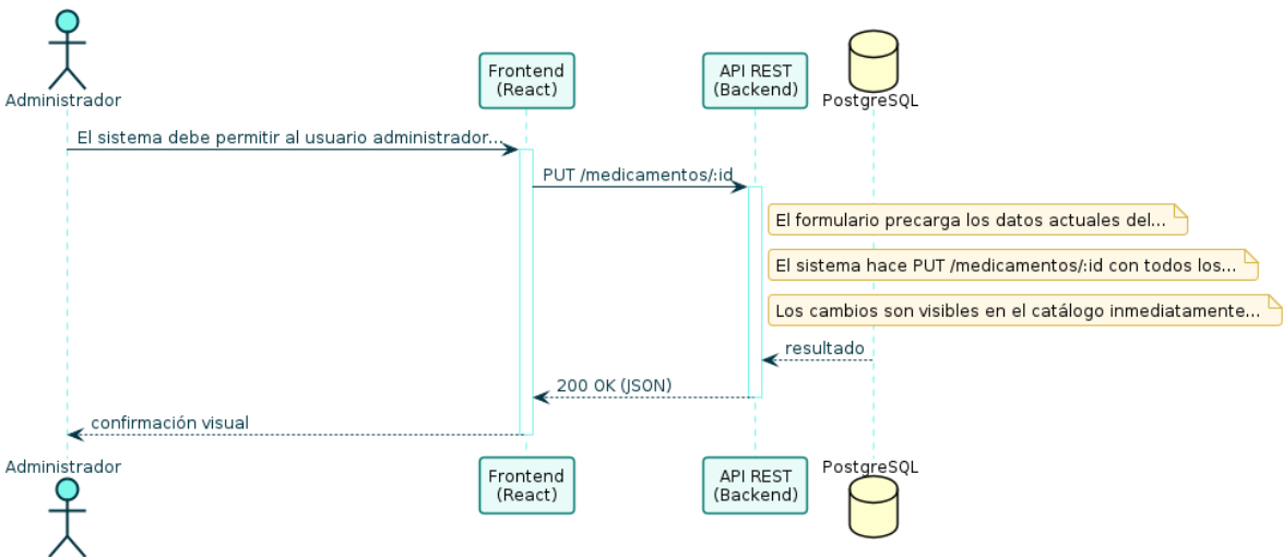
Diagrama de Secuencia — RF-30
