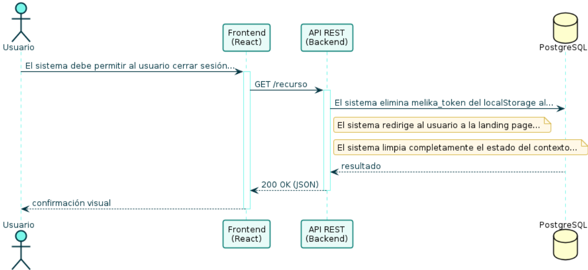
Diagrama de Secuencia — RF-05
