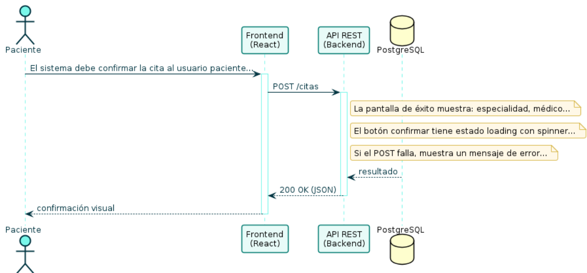
Diagrama de Secuencia — RF-22
