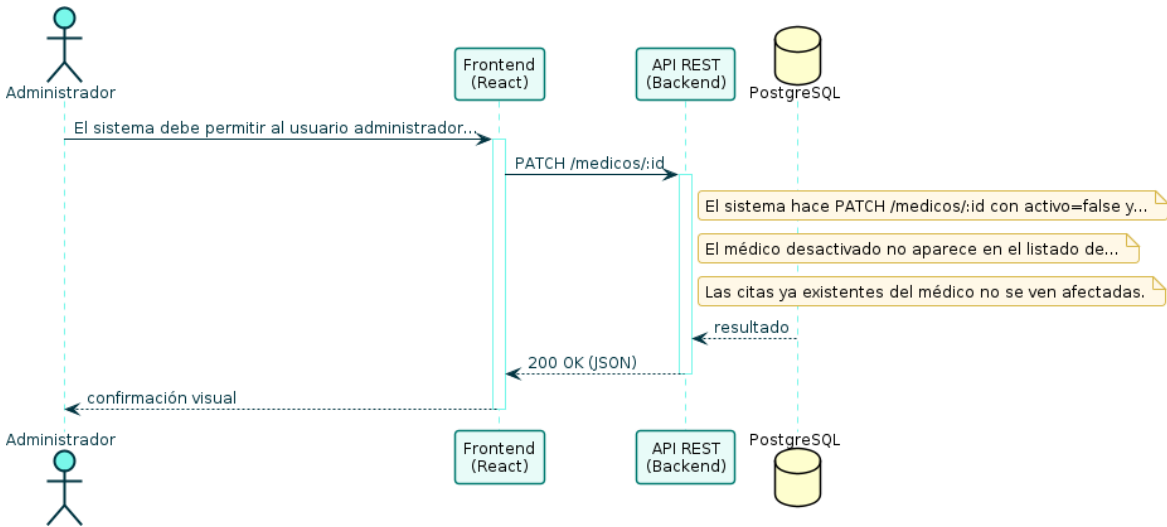
Diagrama de Secuencia — RF-35
