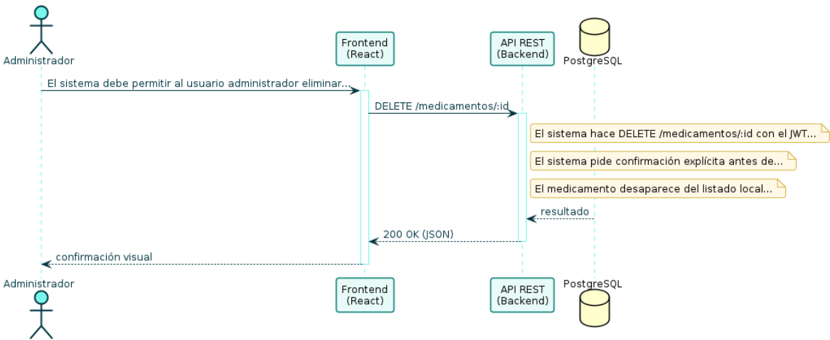
Diagrama de Secuencia — RF-31
