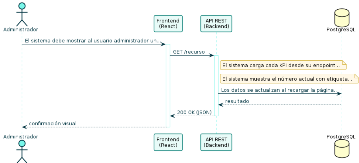
Diagrama de Secuencia — RF-47
