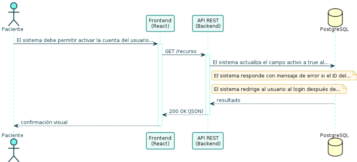
Diagrama de Secuencia — RF-03
